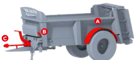
(A) Stalen spatborden (B) Documentenbuis met geïndividualiseerd onderdelenboek (C) Slangenhouder en groothoekaftakas met nokkenbeveiliging.
