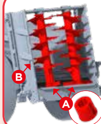
(A) Verwisselbare slijtringen (behalve op 37S08 en 42S09). (B) Gecentraliseerde smeerpunten op de strooiwalsen.
